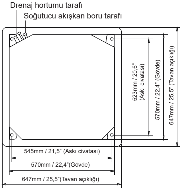
Kompakt modeller tavan deliği boyutu
