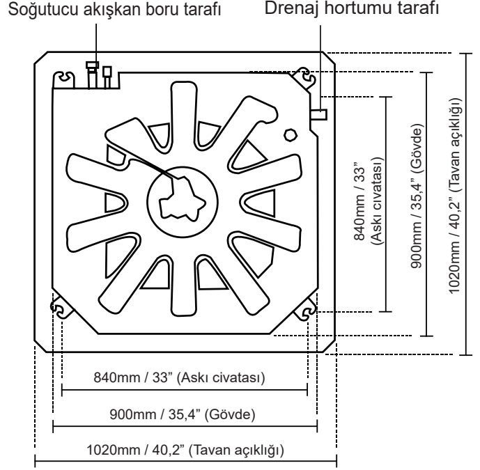
60K Süper İnce modeller tavan deliği boyutu
