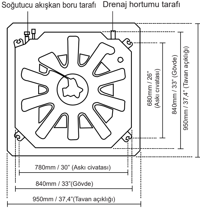
18-48K Süper İnce modeller tavan deliği boyutu
