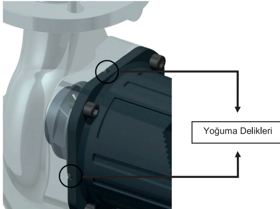
Şekil 6.6: Yoğuşma Delikleri
