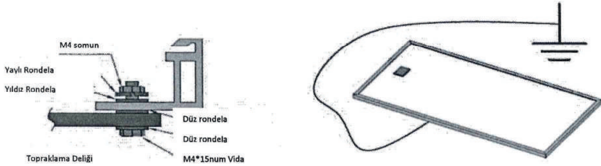
Şekil 4 : Topraklama Grafiği
