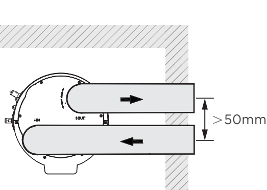
3. L'ingresso dell'aria si collega al condotto, l'uscita dell'aria senza condotti.
