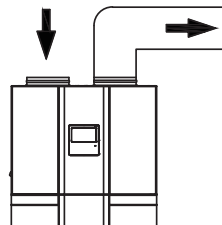
2. Luftauslass verbindet sich mit Kanal, Lufteinlass ohne Kanäle.
