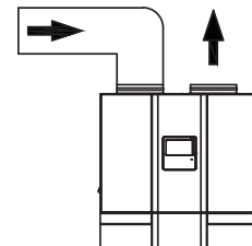
3. Lufteinlass mit Kanal verbunden, Luftauslass ohne Kanäle.
