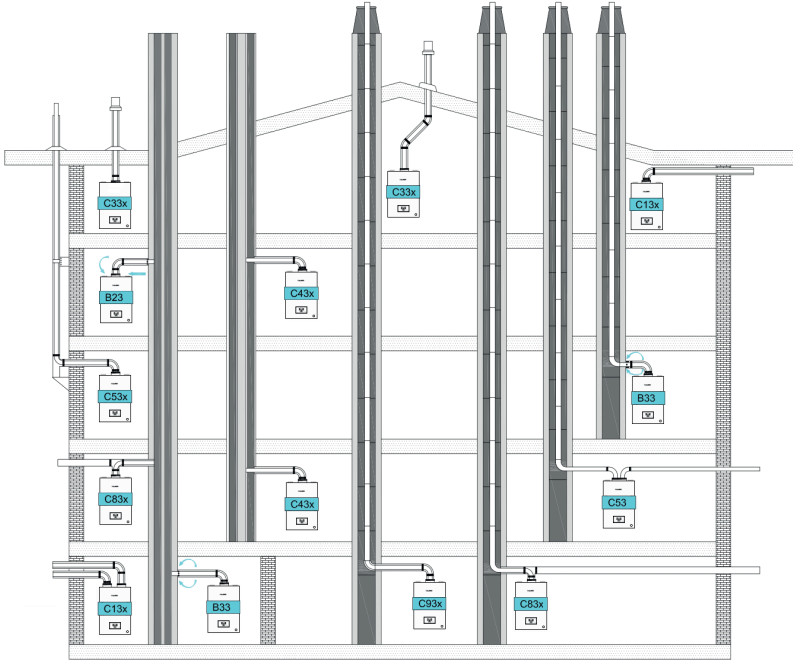
Şekil 24. Baca Uygulamaları
