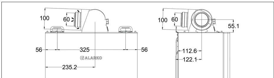
Şekil 27. Ø60/100 mm yatay baca seti ölçüler
