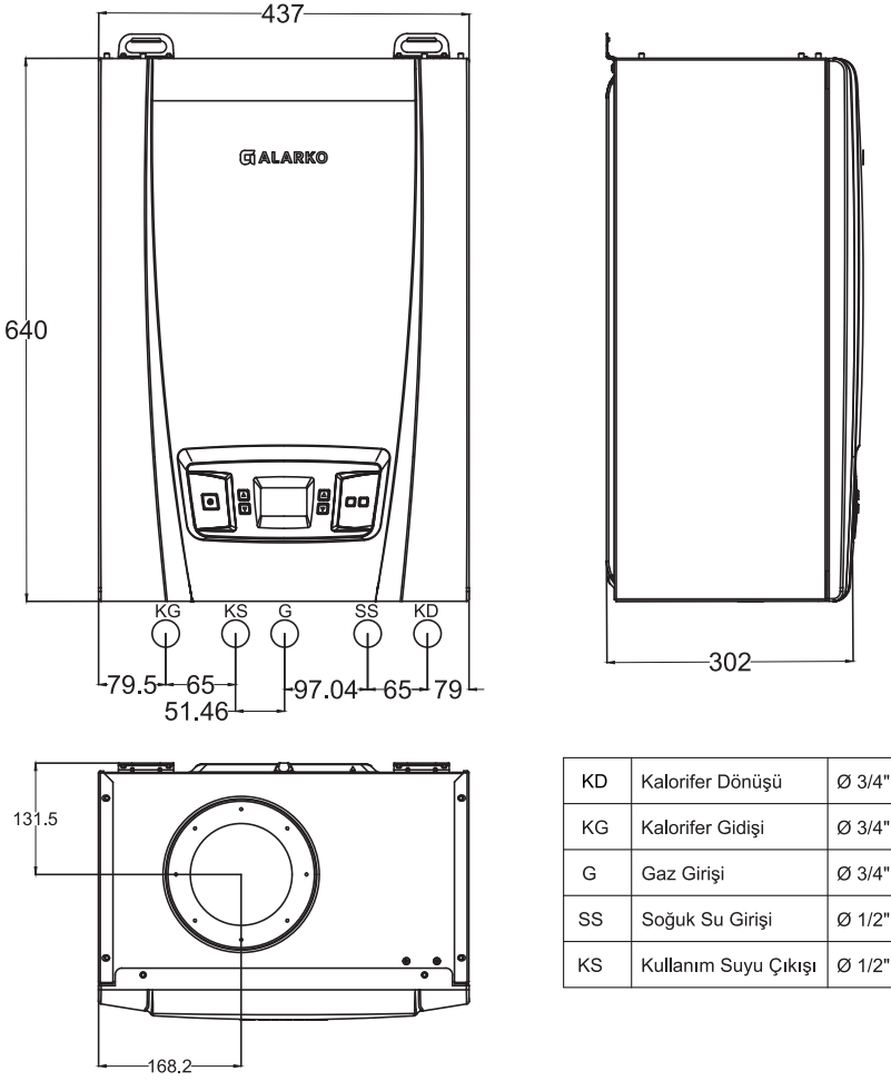
Şekil 5. SSP 20 boyutlar
