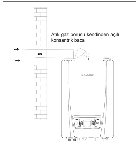
Şekil 21. Konsantrik baca açılıarı
