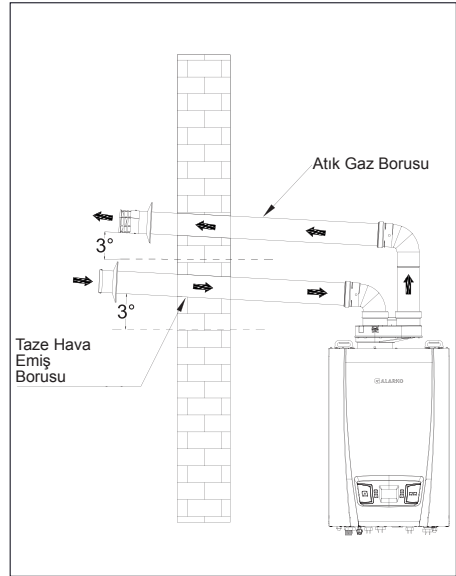
Şekil 20. Hava emiş ve atık gaz boru açılırları
