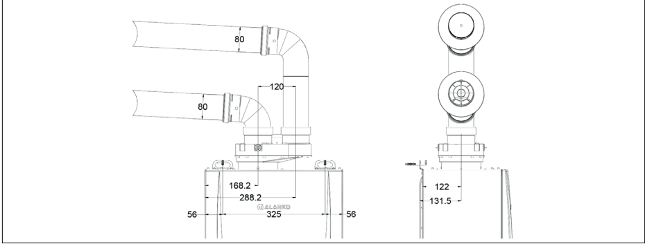
Şekil 28. SRS 20/24/28/36 ikiz baca seti ölçüler
