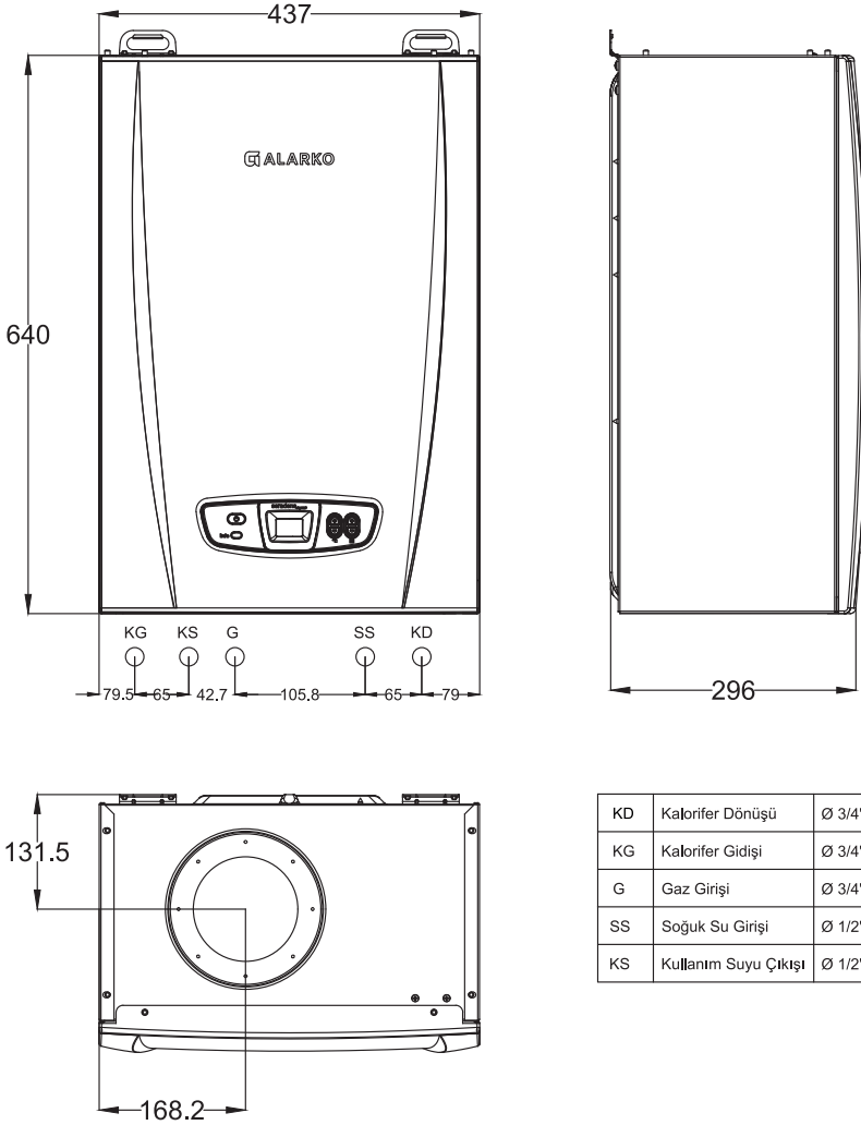
Şekil 5. Boyutlar
