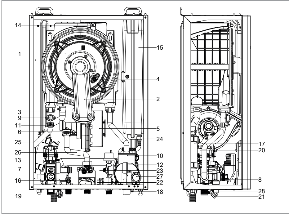
Şekil 7. Ana Parçalar
