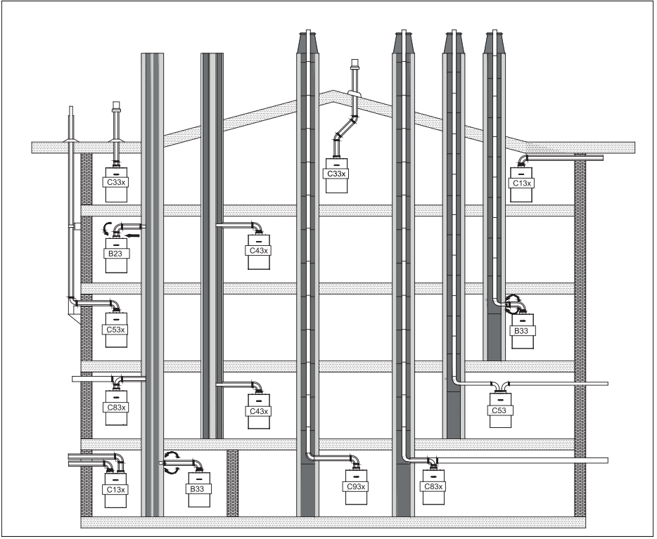
Şekil 24. Baca Uygulamaları
