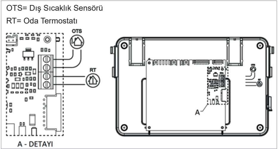
Şekil 19. Plastik panonun iç görünümü
