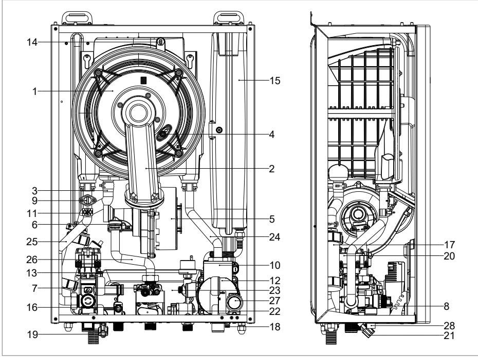
Şekil 7. Ana Parçalar
