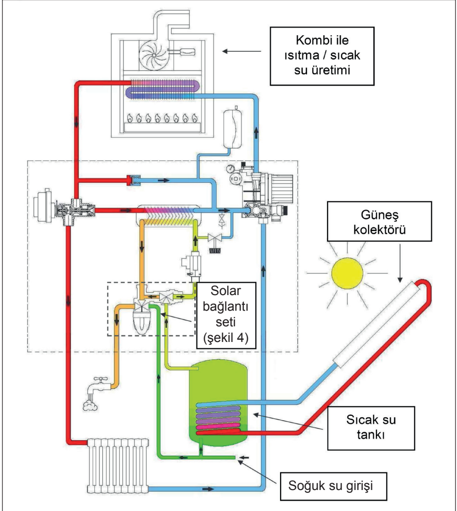
Şekil 3. Solar bağlantı seti uygulaması
