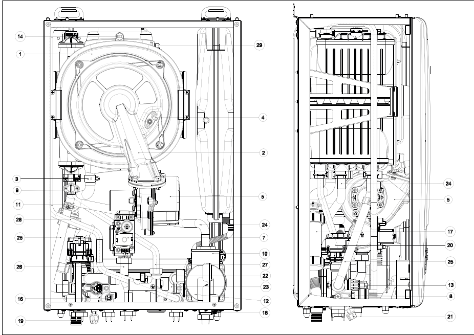
Şekil 7. Ana parçalar
