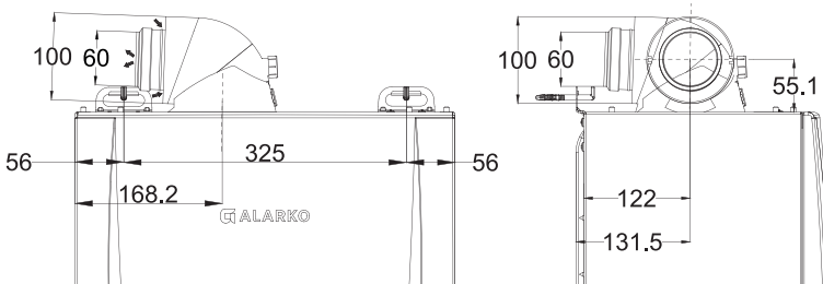
Şekil 27. Ø60/100 mm yatay baca seti ölçüler
