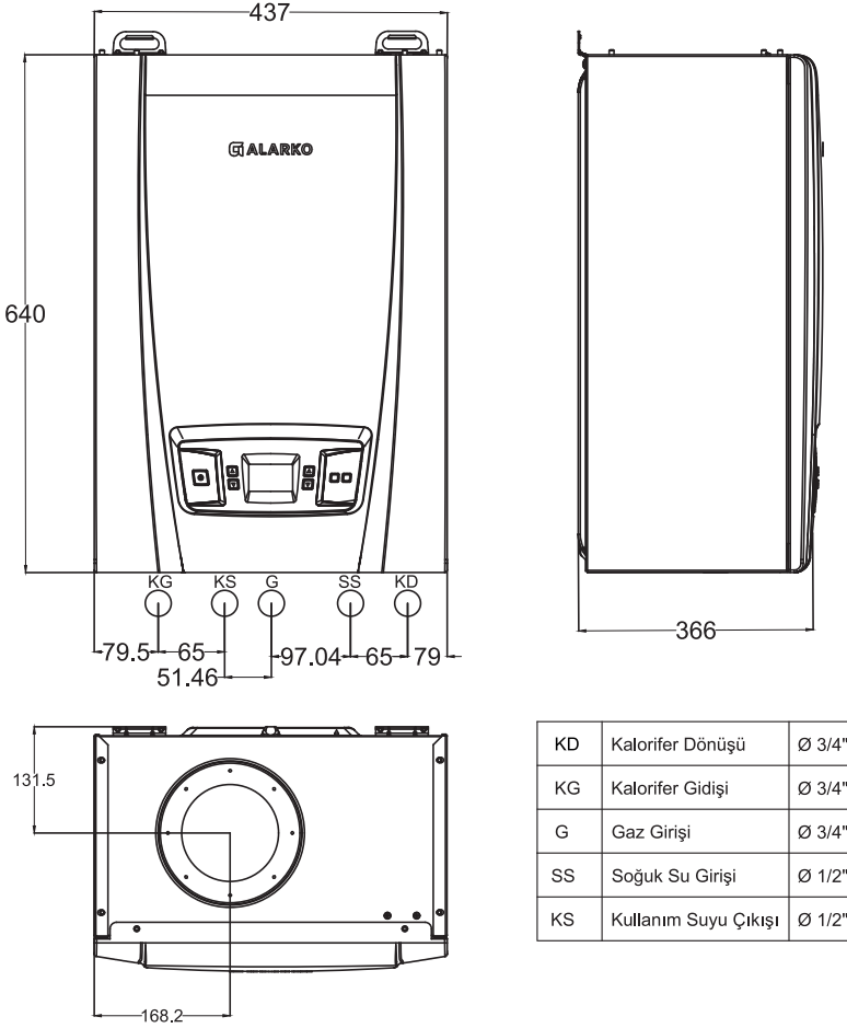
Şekil 6. SSP 24/28/36 boyutlar
