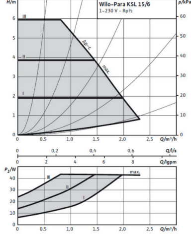
Sabit Basma Yüksekliği Eğrisi (Eğri 2)
