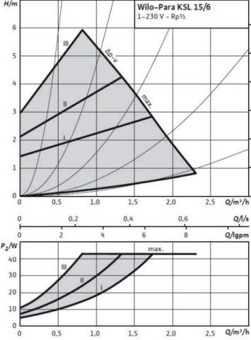
Değişken Basma Yüksekliği Eğrisi (Eğri 1)
