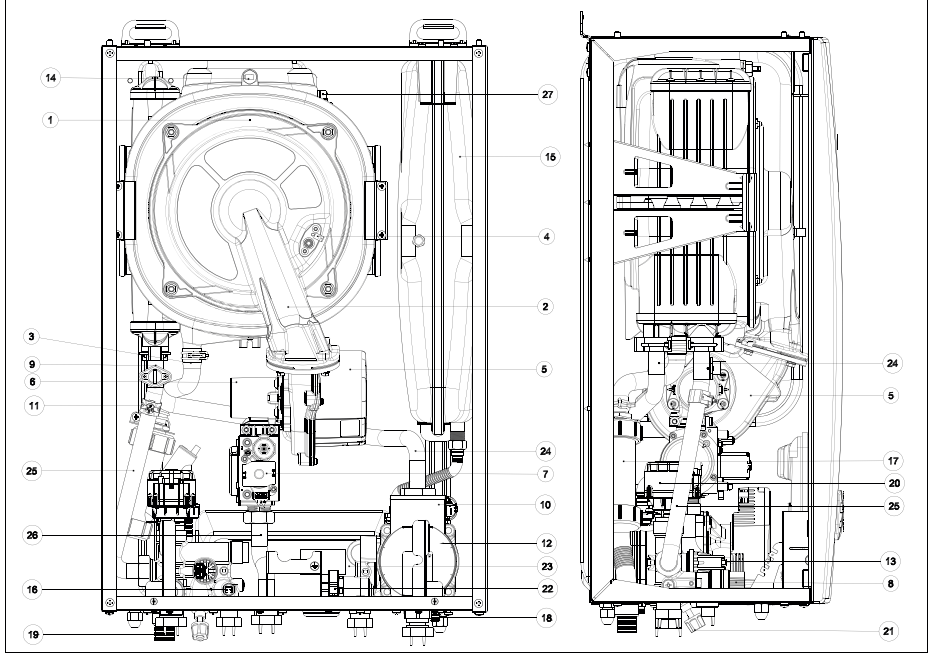
Şekil 6. Ana parçalar
