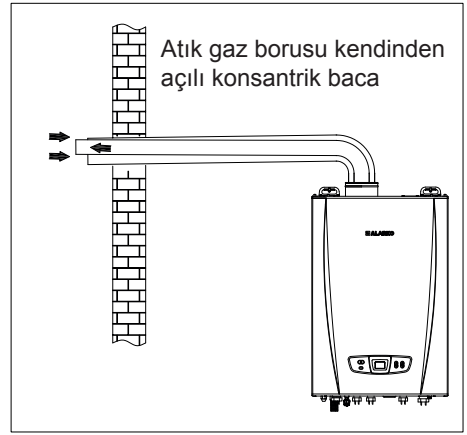
Şekil 20. Konsantrik baca açılı
