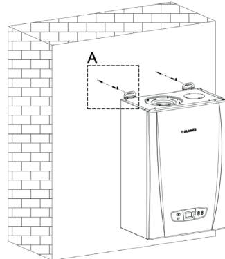
ADIM 2 - MONTAJ
