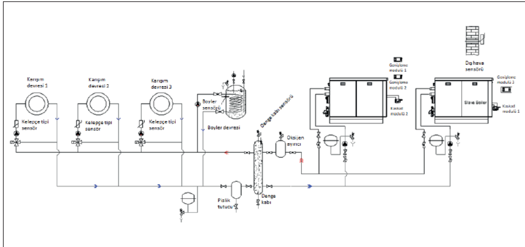
İki (kaskad çalışan) kazan, 3 karışım devresi, 1 boyler devresi bağlantı örneği (denge kabı ile)
