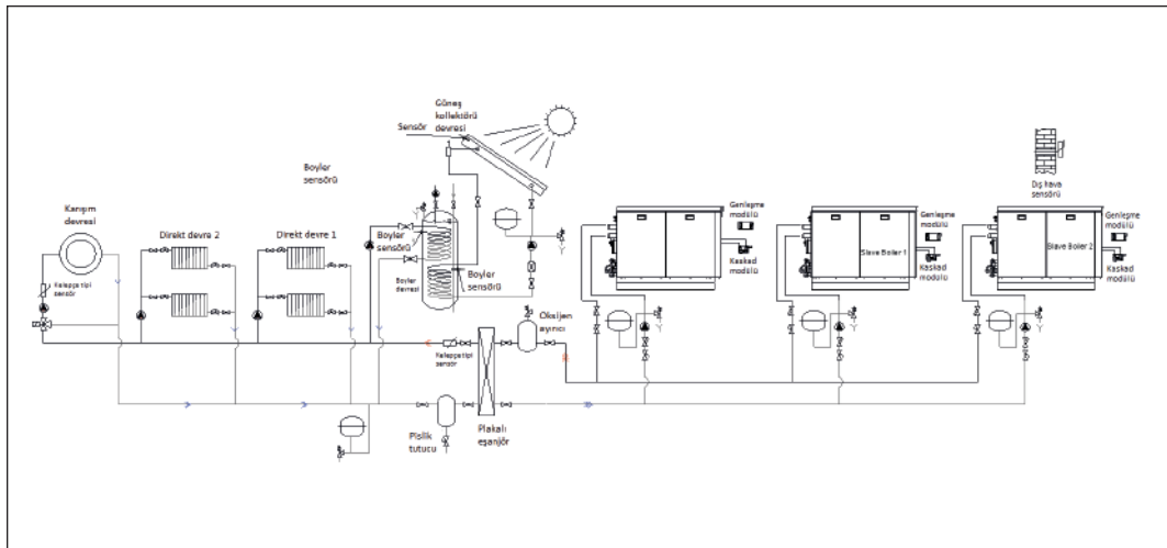
Üç (kaskad çalışan) kazan, 2 direkt devre, 1 karışım devresi, 1 güneş kolektörlü boyler devresinin primer ve sekonder devreyi ayırıcı plakalı eşanjör ile bağlantı örneği
