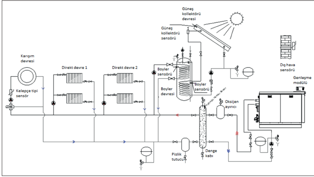
Tek kazan, 2 direkt devre, 1 karışım devresi, 1 güneş kolektörlü boyler devresi bağlantı örneği (denge kabı ile)
