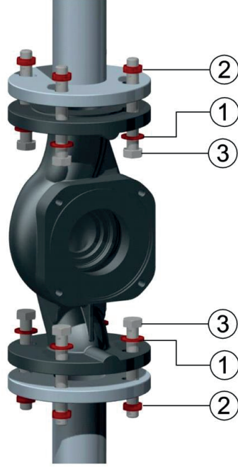
Şekil 6.5: Flanş Bağlantılı Pompa Montajı
