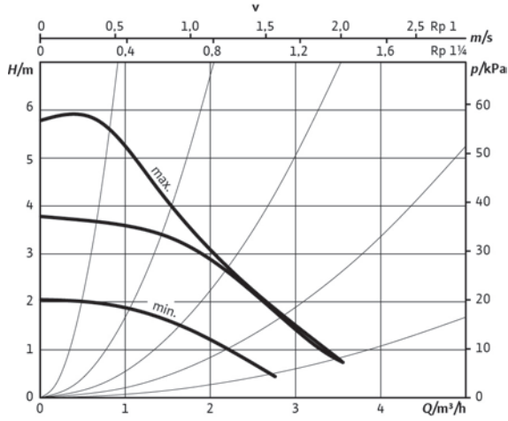
NPVO 25 - 60
