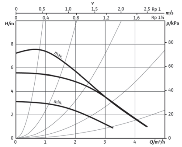
NPVO 25 - 80
