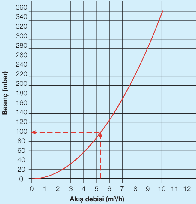
Kazan Basın Kaybı Grafięi
