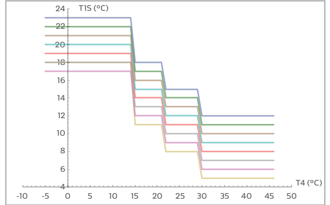
Soğutma Modu İçin Ön Ayar Eğrisi
